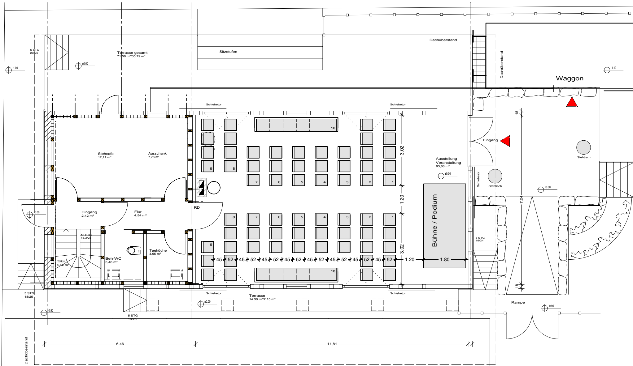
grundriss erdgeschoss
