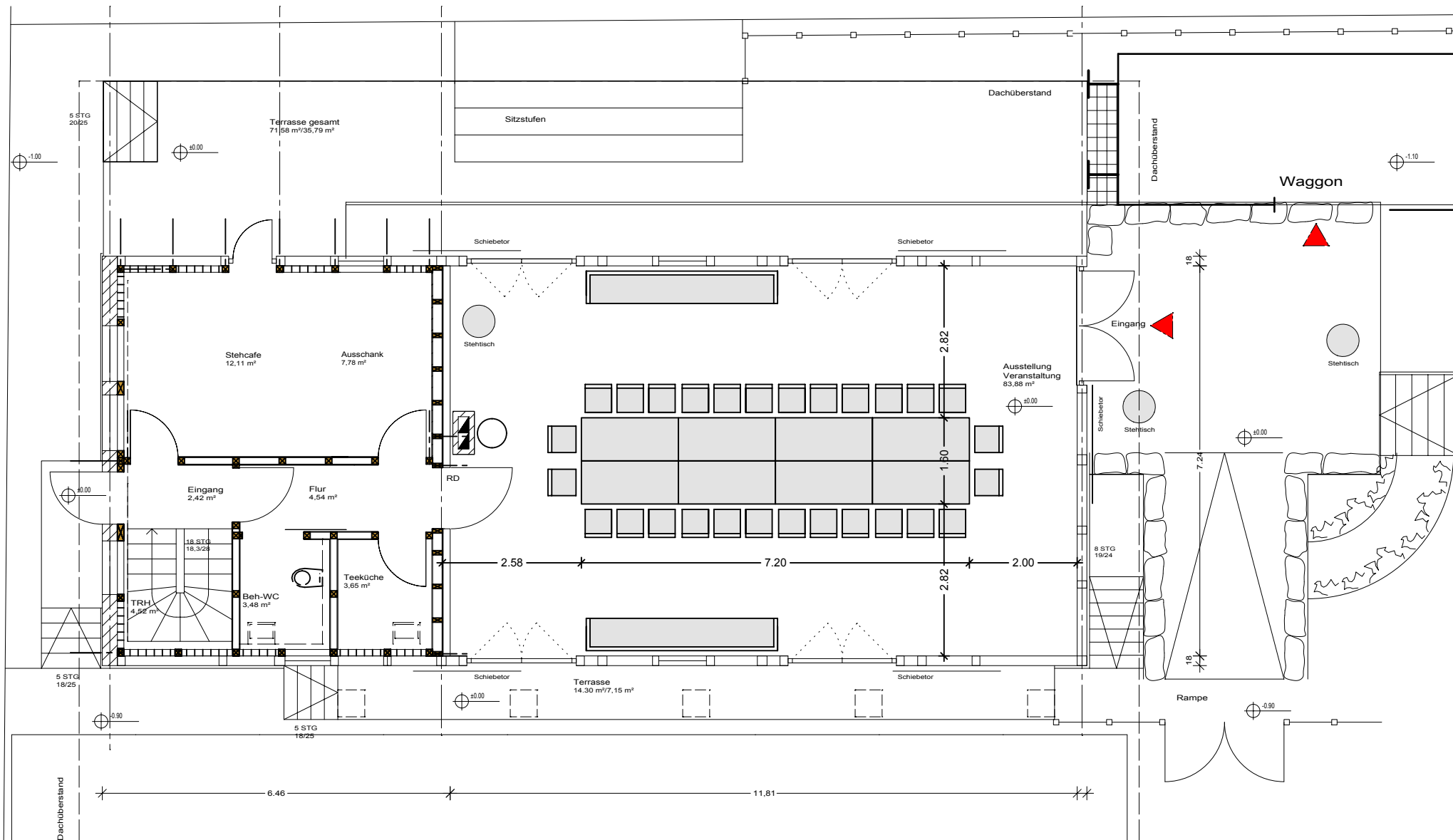
grundriss erdgeschoss
