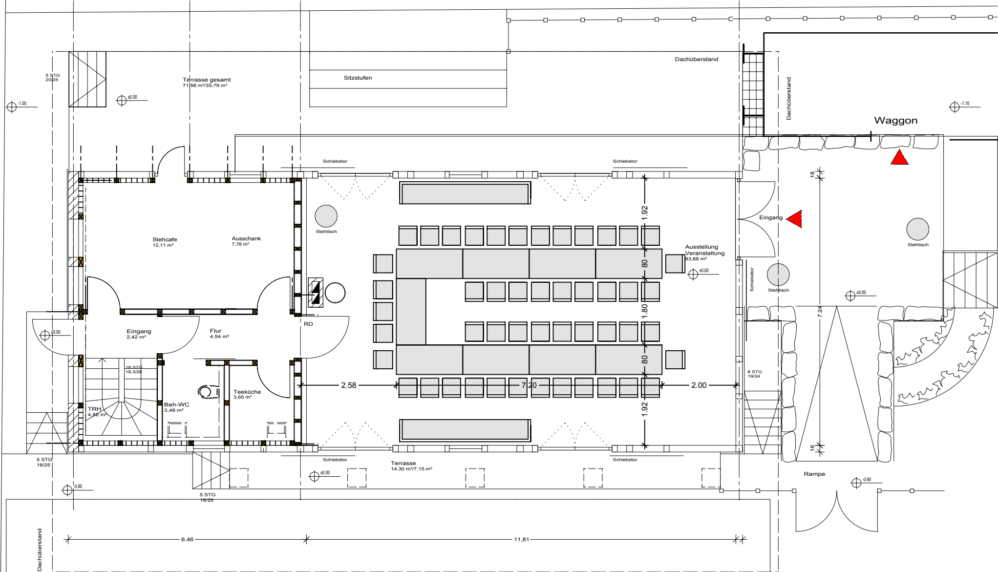
grundriss erdgeschoss
